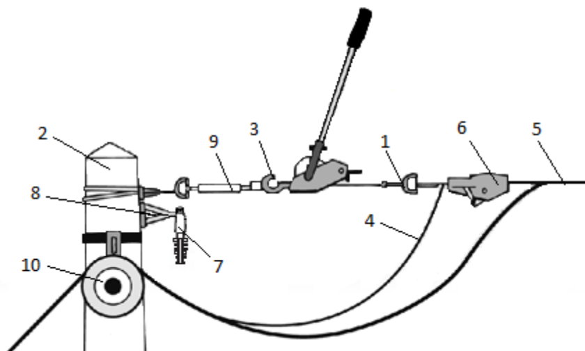
Рис. 2. Схема монтажа СИП с применением ручной лебедки РТ 1000
